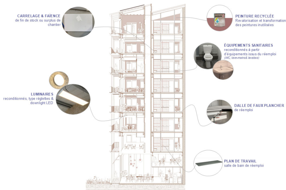
Coupe du bâtiment
